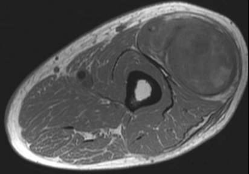
T1強調像
