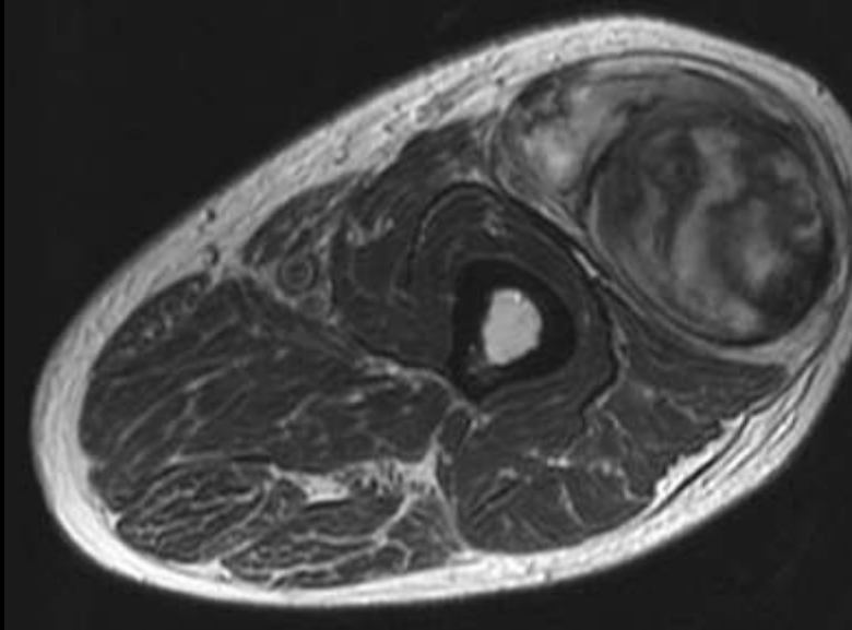
T2強調像
