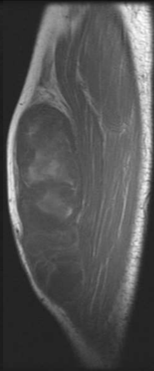
T1強調像
